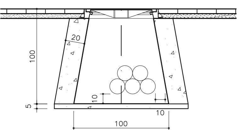
Detalle de arqueta tipo
