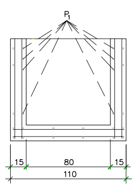
ARQUETA "H" TIPO H-II PARA SITUAR EN ZONAS DE TRAFICO ESPORADICO CALLES PEATONALES O SIN ACERA, APARCAMIENTOS, ETC.
